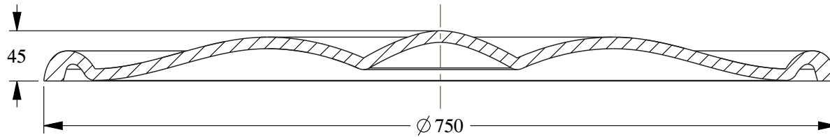
SECTION A-A
